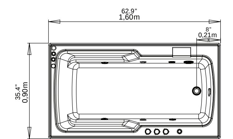
VISTA EN PLANTA / PLANT VIEW
